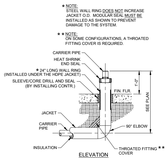
RISER DETAIL SCALE: NONE
