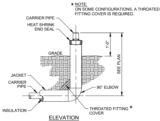
RISER DETAIL SCALE: NONE
